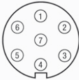
7-Polige Stekker
